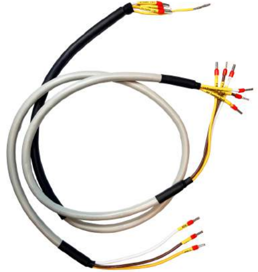
4x4 LIYCY Pano İçi Motor Bağlantı Kabloları 4x4 LIYCY Power Cable Inside Controller
